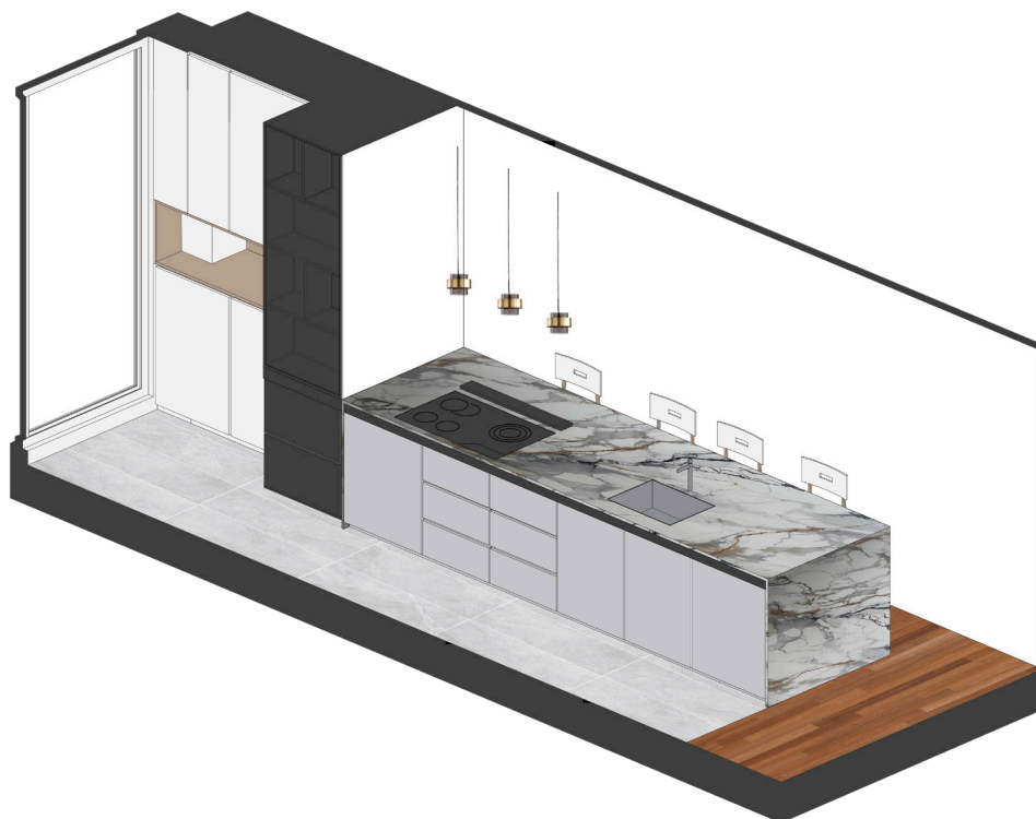
Axonometría - Cocina G&G
