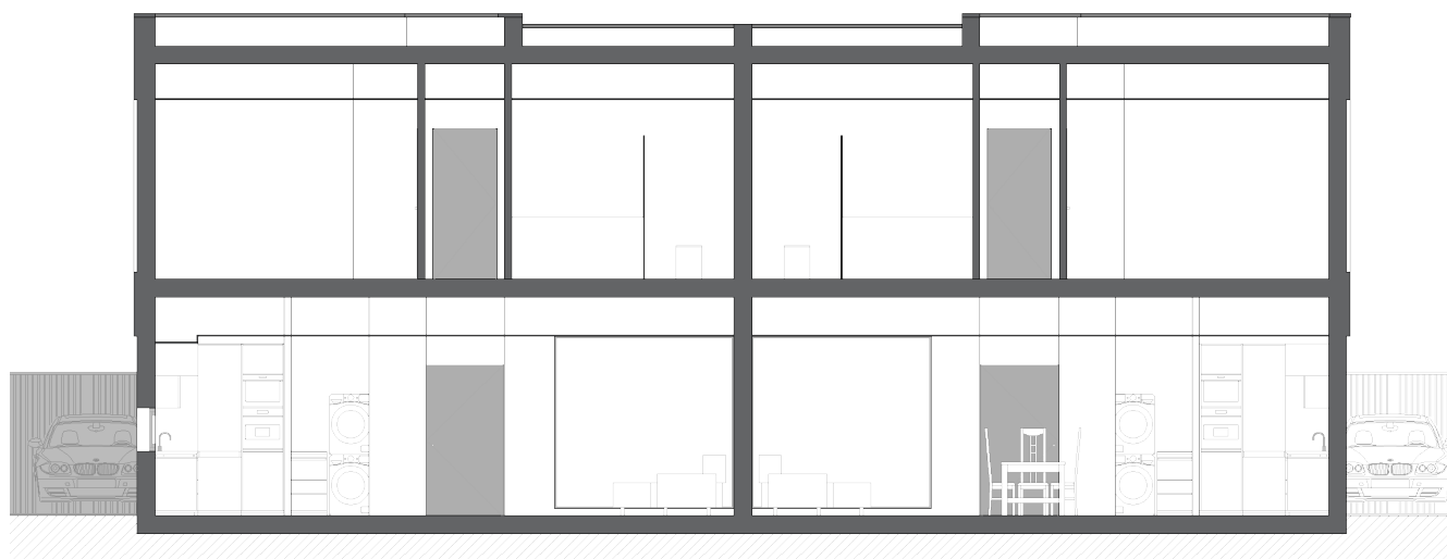
Sección corta - Casa Duo Serra
