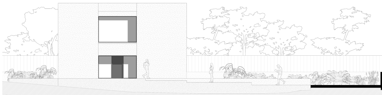
Alzado principal - Casa Magnolia
