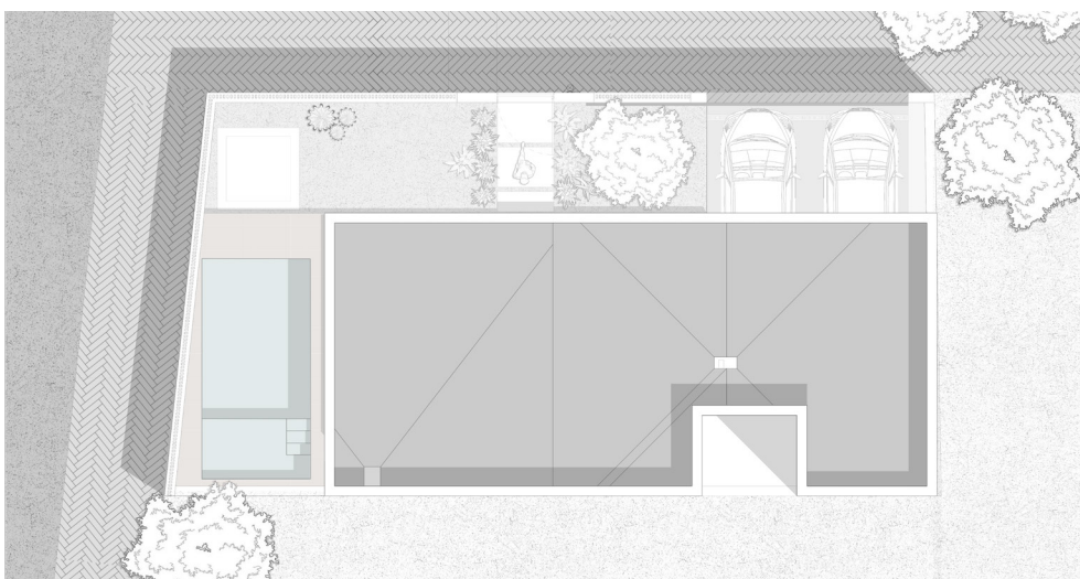
Planta cubierta
