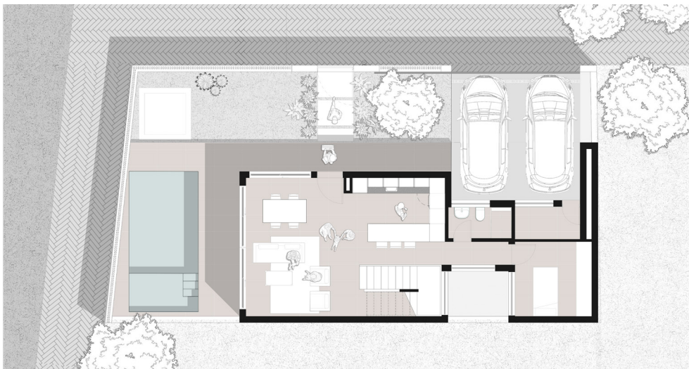
Planta baja
