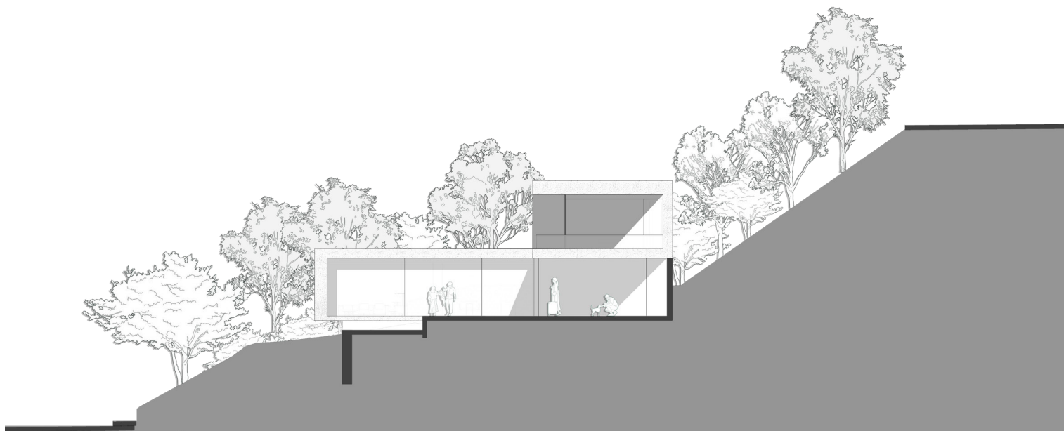
Alzado lateral - Nua House
