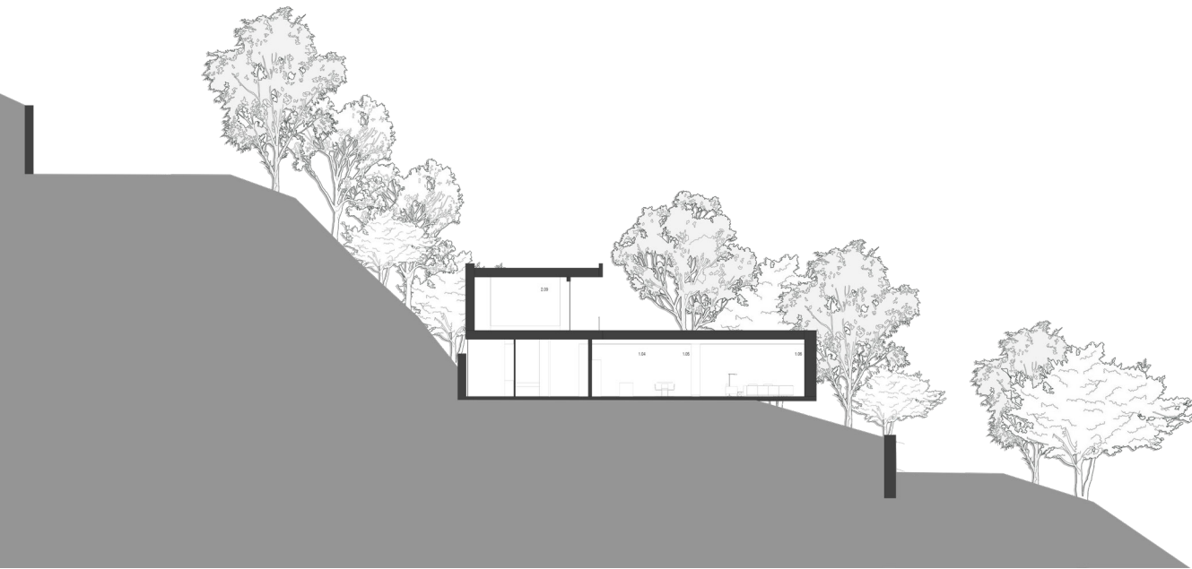
Sección corta - Nua House
