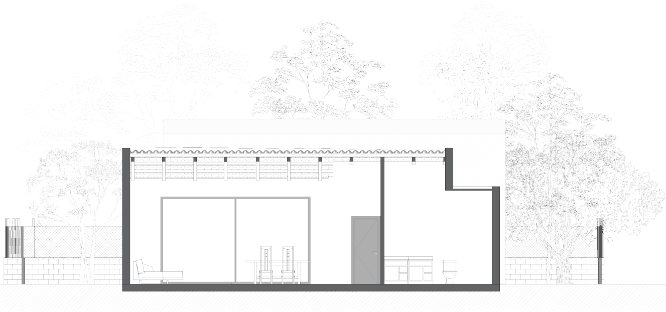
Sección transversal - Casa Guadalupe
