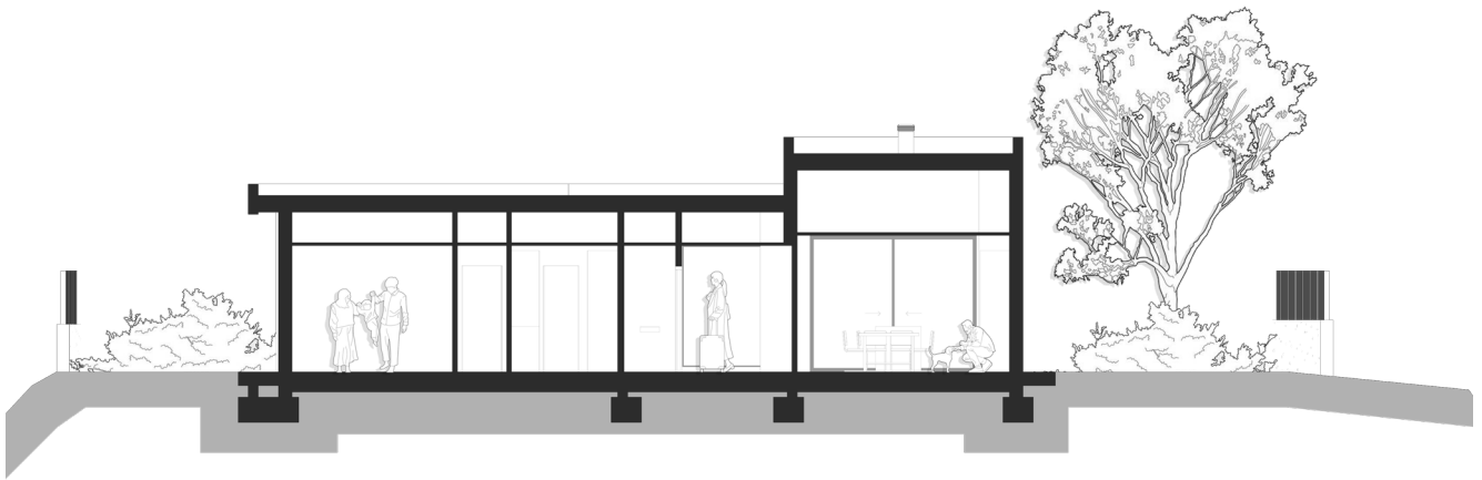
Sección longitudinal - Casa Montemar
