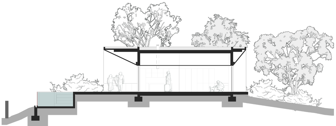
Sección transversal - Casa Montemar
