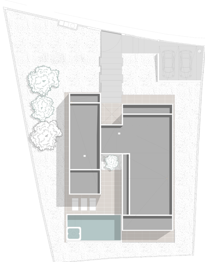
Planta cubierta - Casa Montemar
