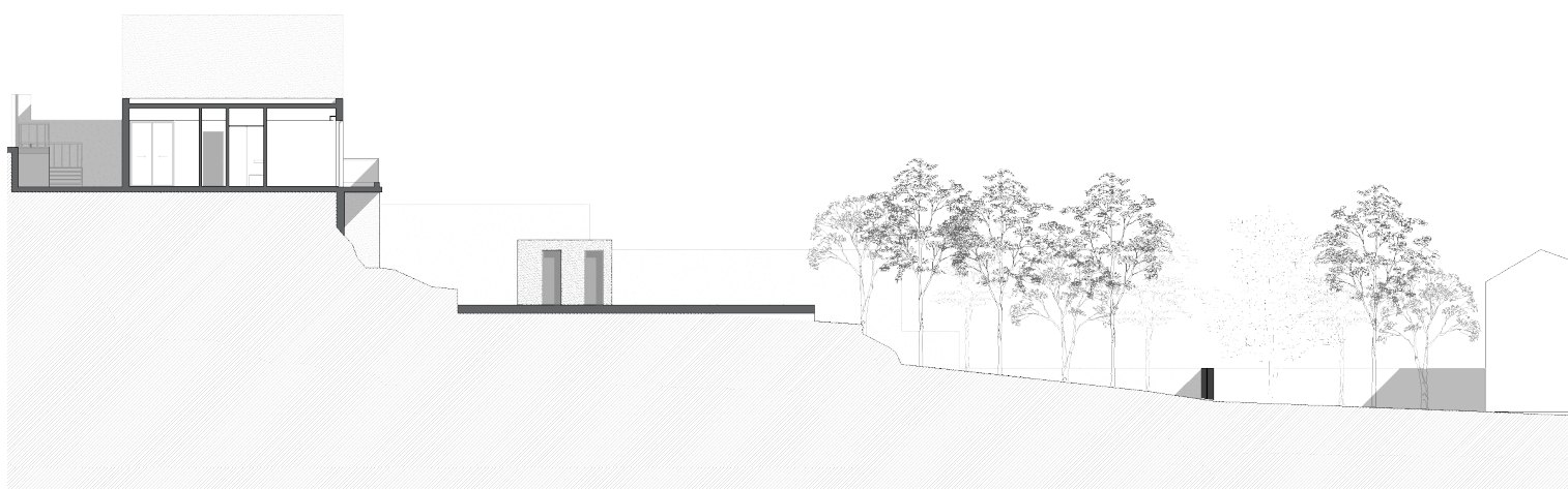
Sección longitudinal - Casa Kairos
