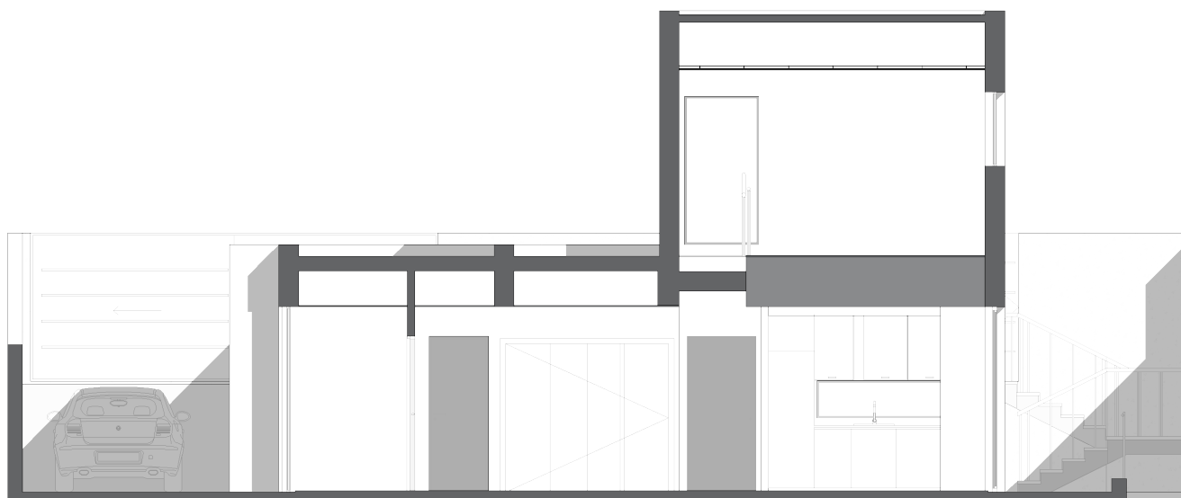
Sección transversal - Casa kairos
