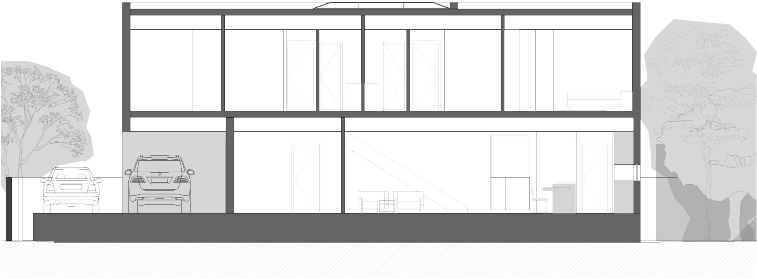
Sección transversal - Casa Cristal
