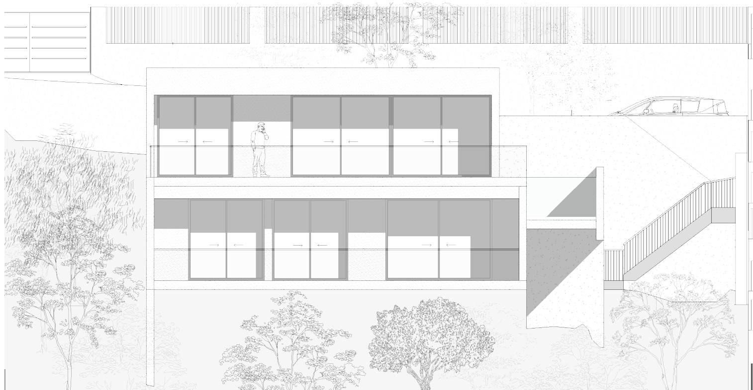
Alzado frontal - Casa Dimale
