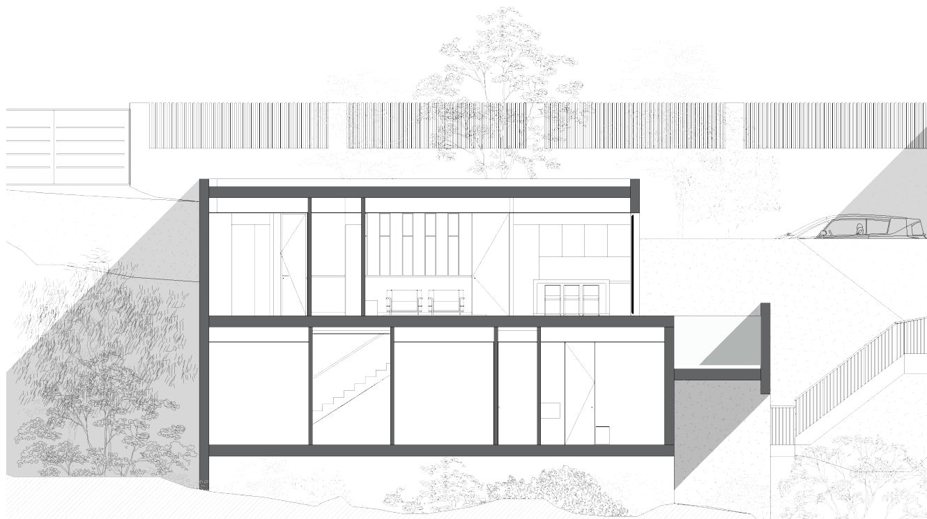
Sección transversal - Casa Dimale
