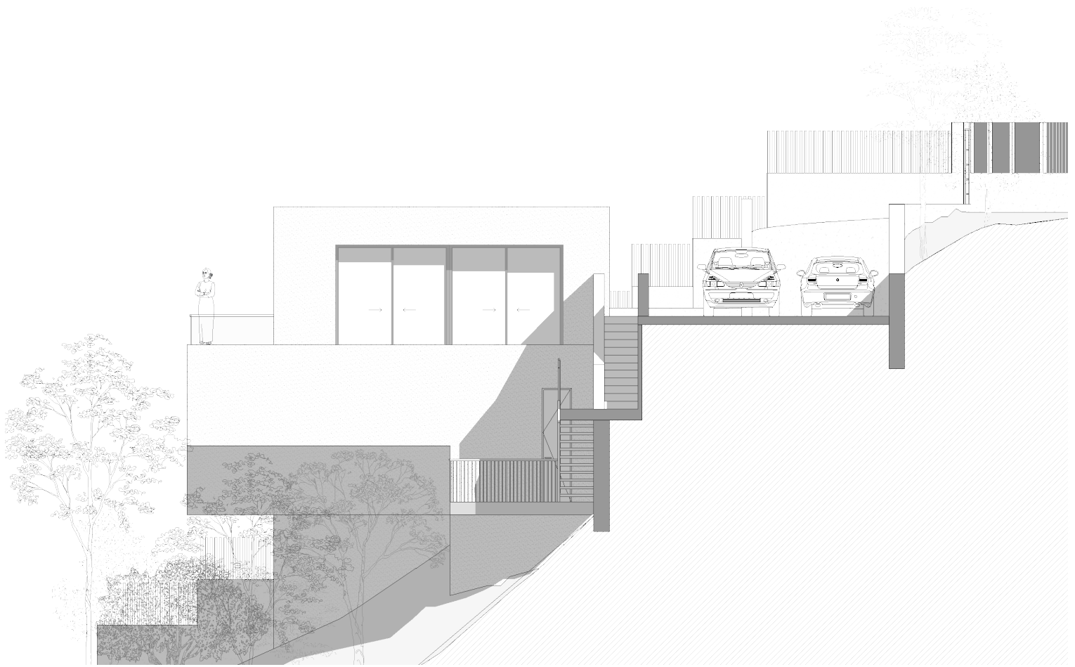
Alzado lateral - Casa Dimale
